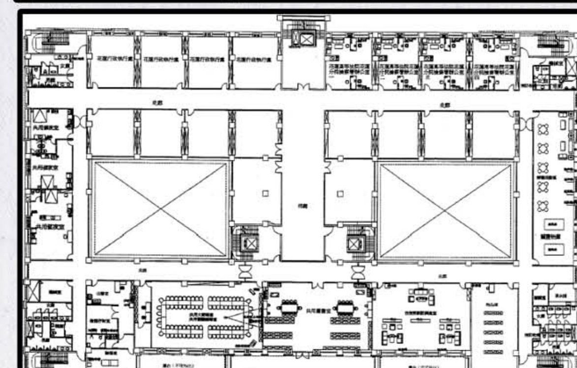
◀ 三層平面圖
