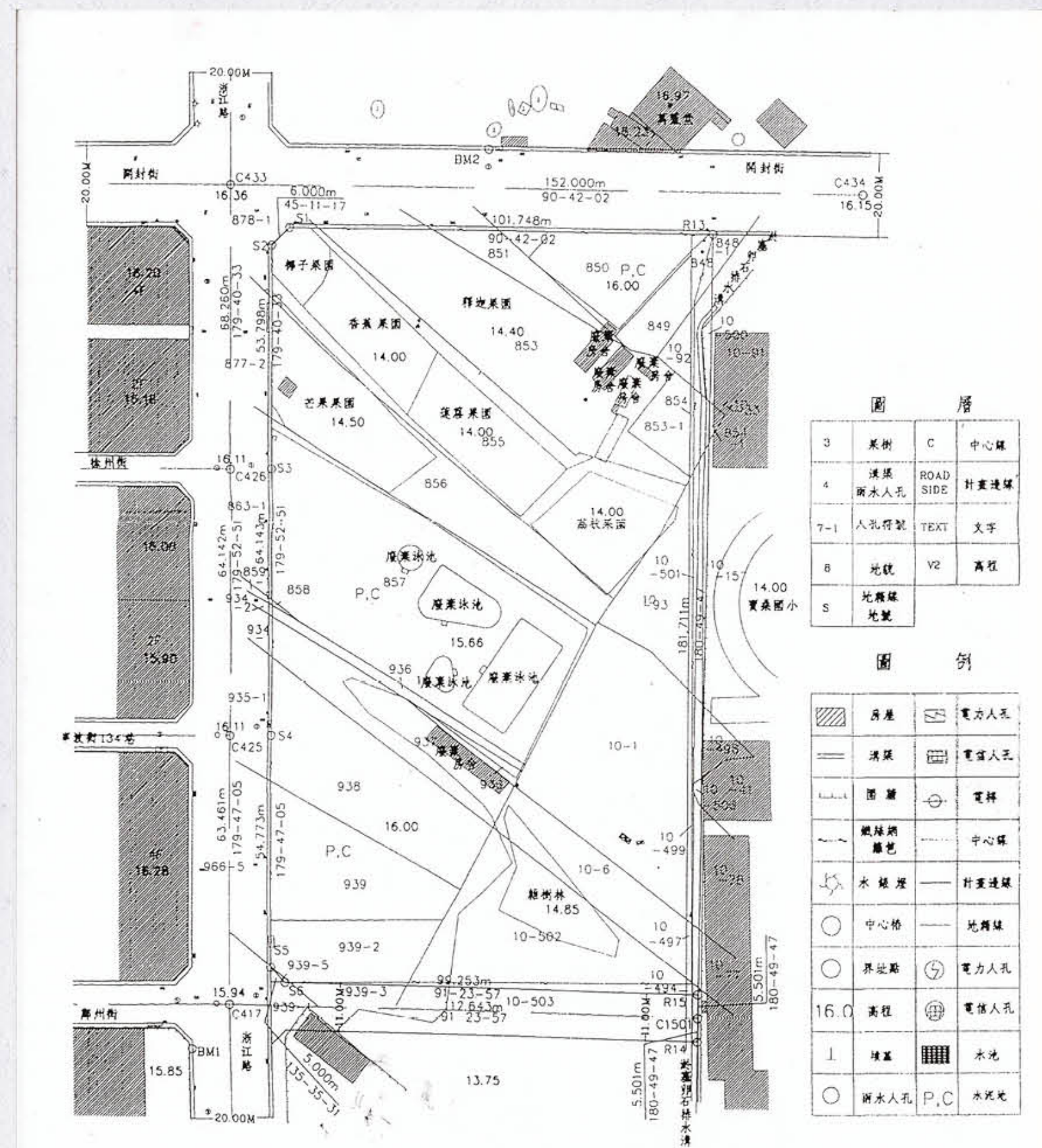
台灣台東地方法院檢察署辦公廳舍地形圖 比例尺：一千分之一
