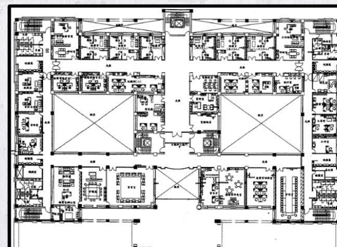
◀ 二層平面圖
